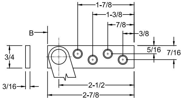
JAMB BRACKET
